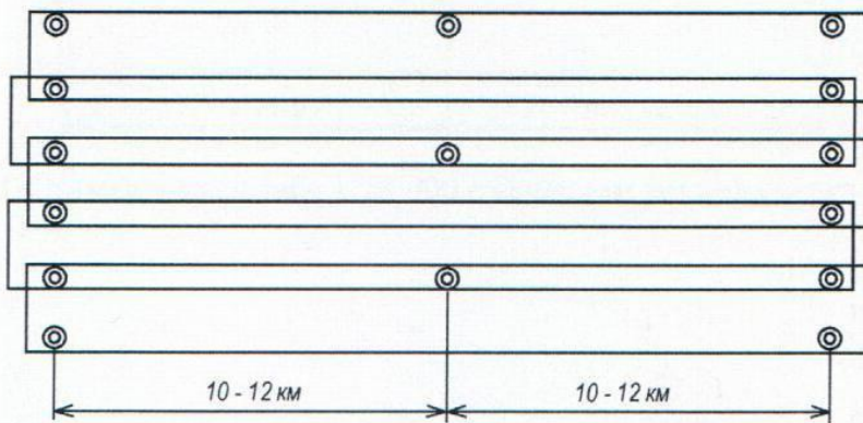
Рис. 5. Съемка в масштабе 1:10 000 с сечением рельефа через 5,0 м
