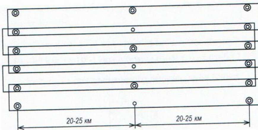
Рис. 7. Съемка в мащтабе 1:25 000 с сечением релъефа чрез 5,0 м
