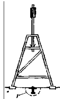
Рис. 30. Пирамида-штатив со съемной визирной целью 1 - марка триангуляционная
