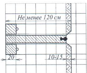
Чертеж нового центра и размеры
