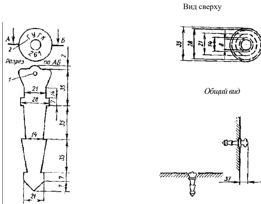
Рис. 37. Стенной знак пункта полигонометрии 2, 3, 4 классов, 1 и 2 разрядов. Тип 8 г. р. 1 - отверстие диаметром 2 мм для установки визирного приспособления; 2 - надпись, состоящая из начальных букв организации, производящей геодезические работы.
