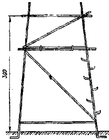
Рис. 27. Металлическая переносная площадка для наблюдения с пирамид-штативов. Изготавливается из уголковой стали (50x50x5 и 35x35x4)
