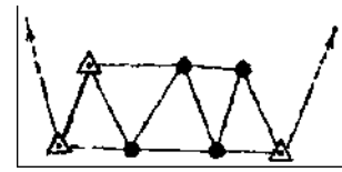
Рис. 23 Цепочка треугольников между стороной и пунктом
