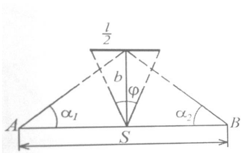
Рис. 13 S_{AB} = l/2 \operatorname{ctg} \varphi/2 (\operatorname{ctg} \alpha_1 + \operatorname{ctg} \alpha_2)
