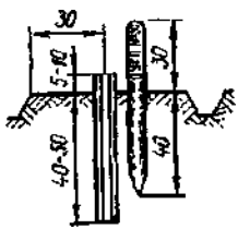
Рис. 45 Металлическая труба, кованый гвоздь со сторожкой
