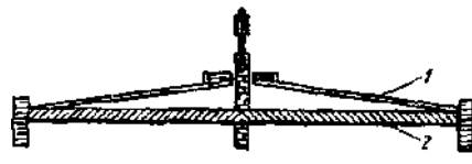
Рис. 29. Тур со съемной визирной целью 1 - крыша; 2 - перекрытие (балка)
